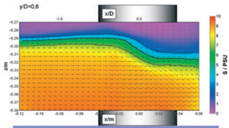
Geschwindigkeitsfeld und Salinität neben dem Zylinder, gemessen mit PLIF/PIV im Kanal für geschichtete Strömungen. Deutlich ist der Einfluss des Fundamentmodells auf den Verlauf der Salzwasserströmung und der Mischungsschicht ersichtlich (Abb. 4).
