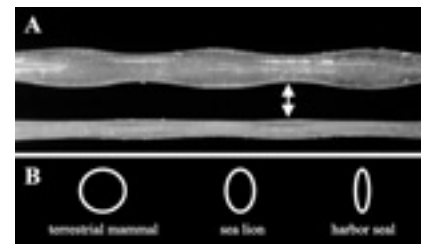
Das Barthaar des Seehundes aus der Familie der Hundsrobben hat eine wellige Längsstruktur (A) und einen ovalen Querschnitt, im Gegensatz zum Barthaar von Landsäuern oder Seelöwen (B) (Abb. 3).
